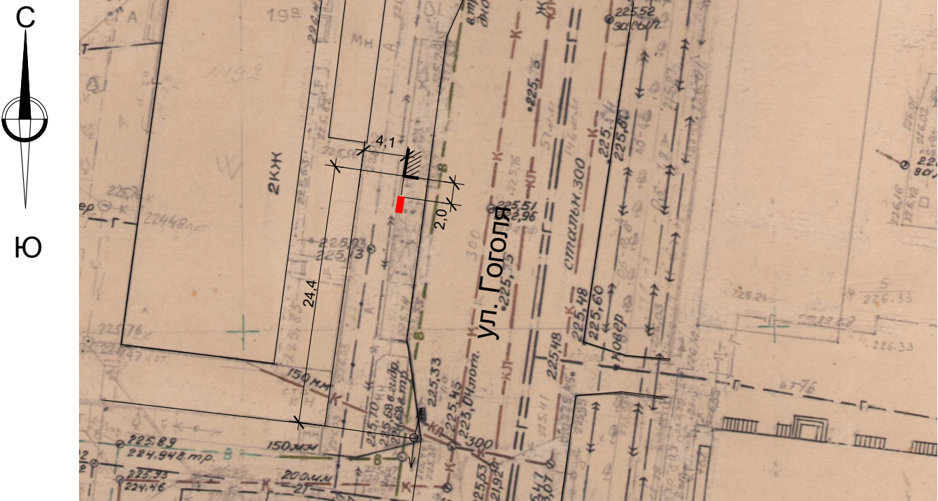
Карта - схема размещения рекламной конструкции №6 М 1:500
